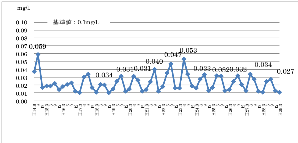
図-4 丸尾平配水池の総トリハロメタンの推移
