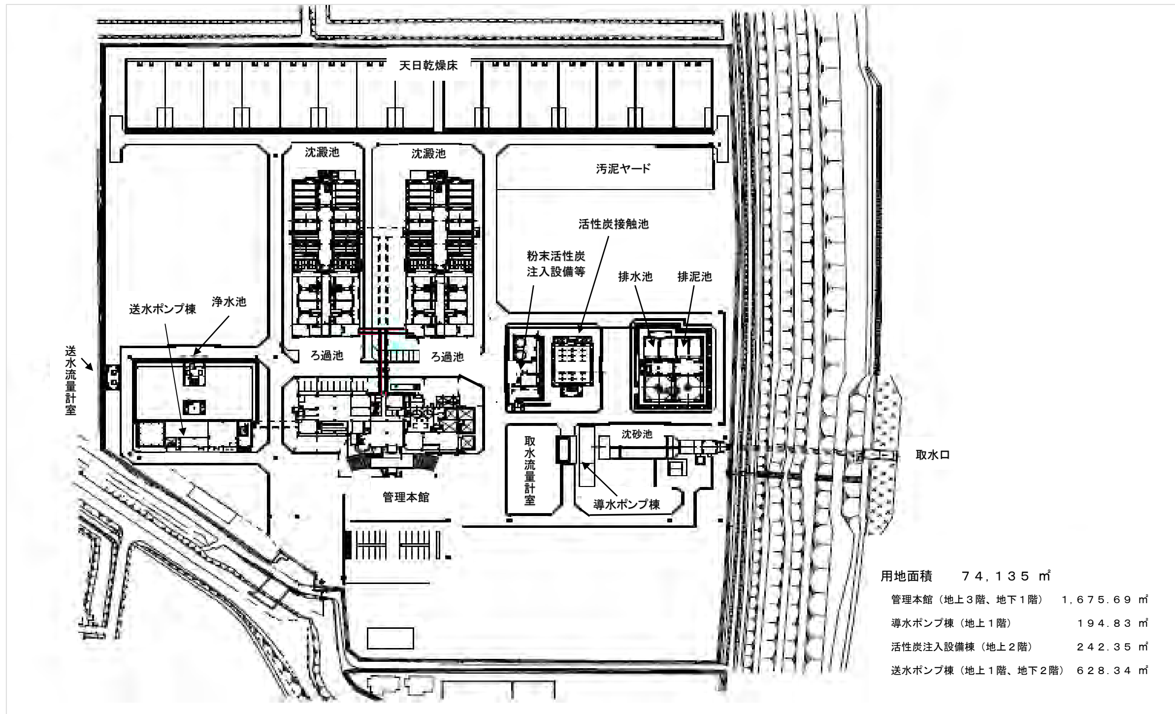
ア 嘉瀬川浄水場平面図
