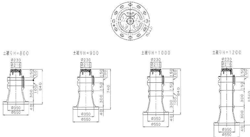
図5-3 仕切弁ボックス仕様図
