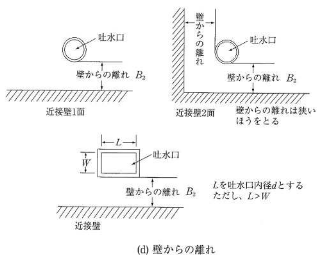
図6-6 基準省令に規定する吐水口空間
