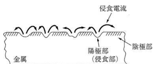
図6-4 ミクロセル浸食の概要図
