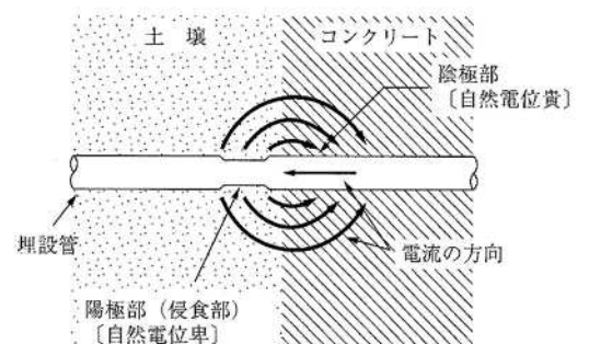
図6-5 コンクリート/土壌系による腐食
