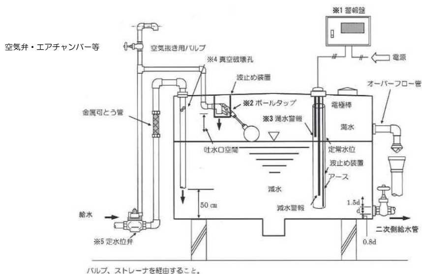
図9-7 受水槽内部構造及び警報設置例（定水位弁・ \phi 25\text{mm} \sim \phi 30\text{mm} ）
