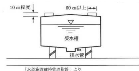
図9-3 マンホール及び排水管の設置
