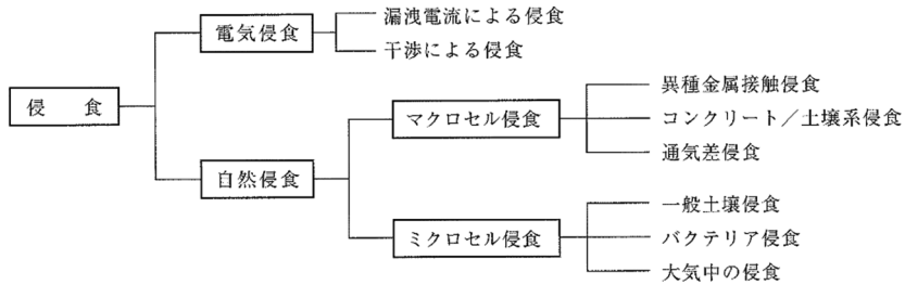
図6-1 腐食の種類
